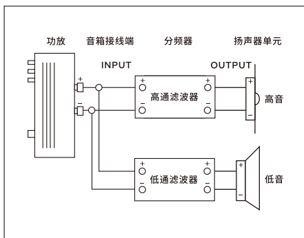
接线图
